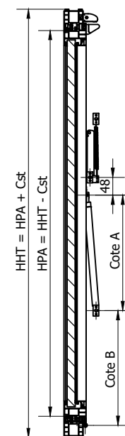
A-A ( 1:10 )
