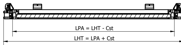
B-B ( 1:10 )
